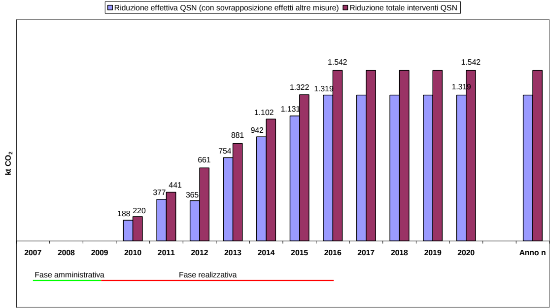
Figura III.2 Efficienza energetica: scenari di impatto sulle emissioni di gas a effetto serra degli investimenti FESR (t in migliaia di CO 2 annue)
